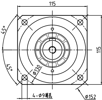
输出端 (Output)
