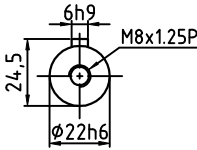
轴型式 S2
