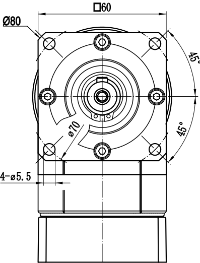
输出端 / OUTPUT
